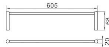
Model: YS-30011 Towel rail 毛巾架
