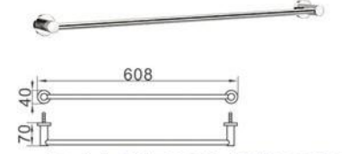
Model: BW-68240 / BW-68300 Towel rail Size: 60cm / 70cm 毛巾架
