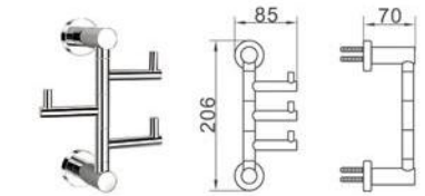
Model: BW-68540C Swivel triple robe hook 三層活動衣帽鉤
