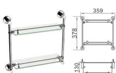
Model: BW-68020 Double glass shelf 雙層置物架
