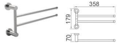
Model: BW-68120 Swivel double towel rails 二層活動杆
