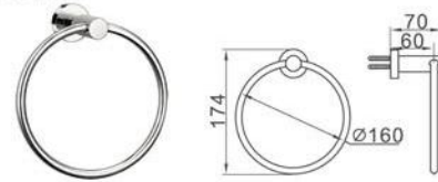
Model: BW-68600 Towel ring 毛巾環
