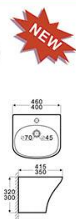
JH-5100C/JH-5100D 半柱盆 尺寸: 460x415x320 毫米 尺寸: 400x350x300 毫米 Half Pedestal Basin Size: 460x415x320mm Size: 400x350x300mm
