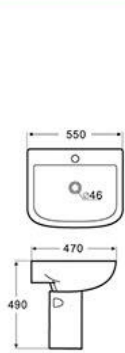
BLT-2004G 半柱盆 尺寸: 550x470x490 毫米 Half Pedestal Basin Size: 550x470x490mm
