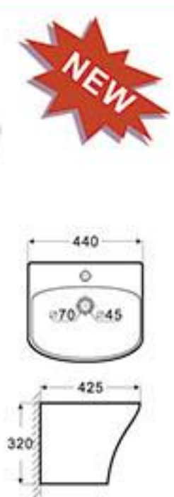
JH-5200C 半柱盆 尺寸: 440x425x320 毫米 Half Pedestal Basin Size: 440x425x320mm
