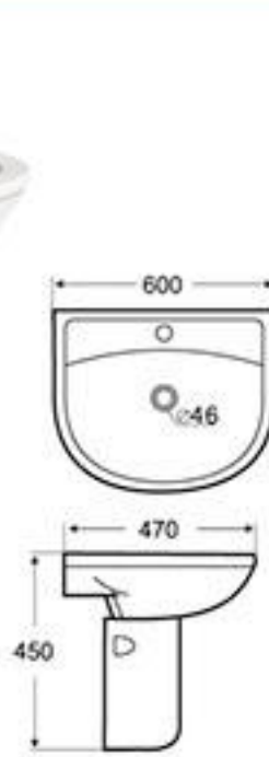
BLT-302G 半柱盆 尺寸: 600x470x450 毫米 Half Pedestal Basin Size: 600x470x450mm
